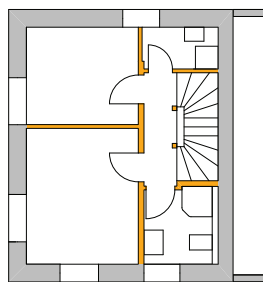
1. Obergeschoss
