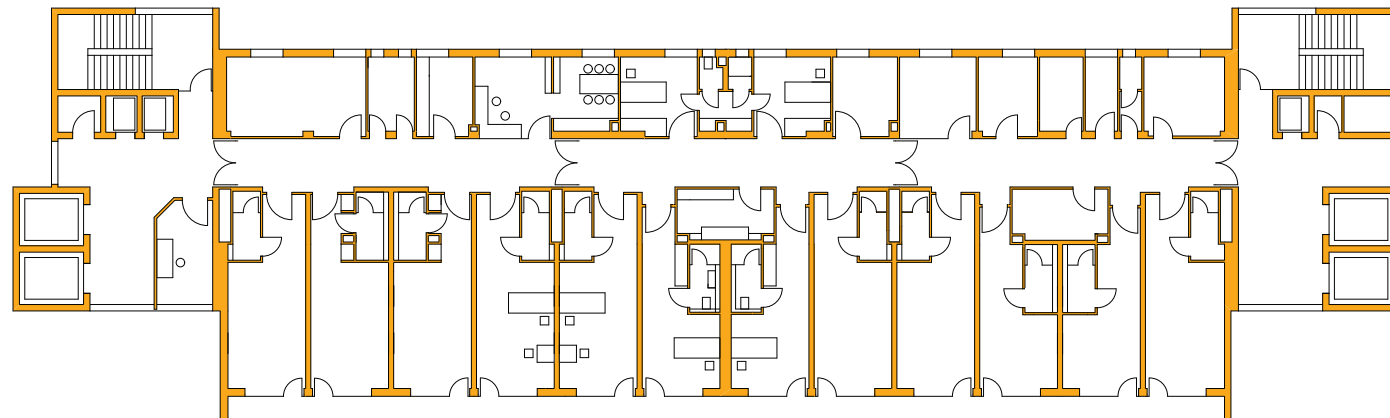
7. Obergeschoss
