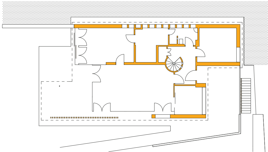
Erdgeschoss
